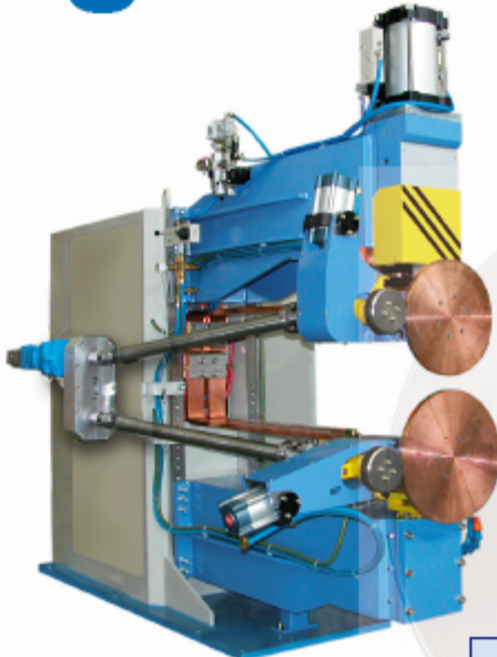
Gamma 314 con doble tracción periférica.
